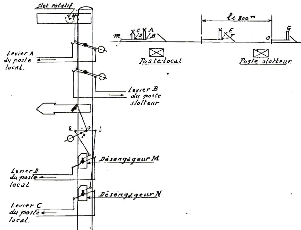
Fig. 110. — Schéma de la manœuvre d'une palette d'arrêt absolu à trois positions conjuguée avec une palette avertisseur à trois positions répétant les indications de deux signaux situés en aval et distants l'un de l'autre de moins de 800 m.
