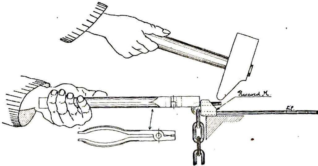
Fig. 57. — Pince servant à tenir la boucle au moment du rabattement.
