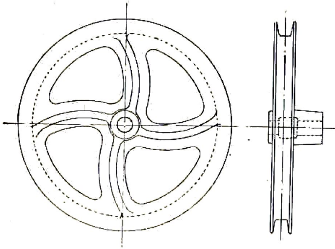
Fig. 39. — Poulie de renvoi de 300 mm. de diamètre pour chaînette.
