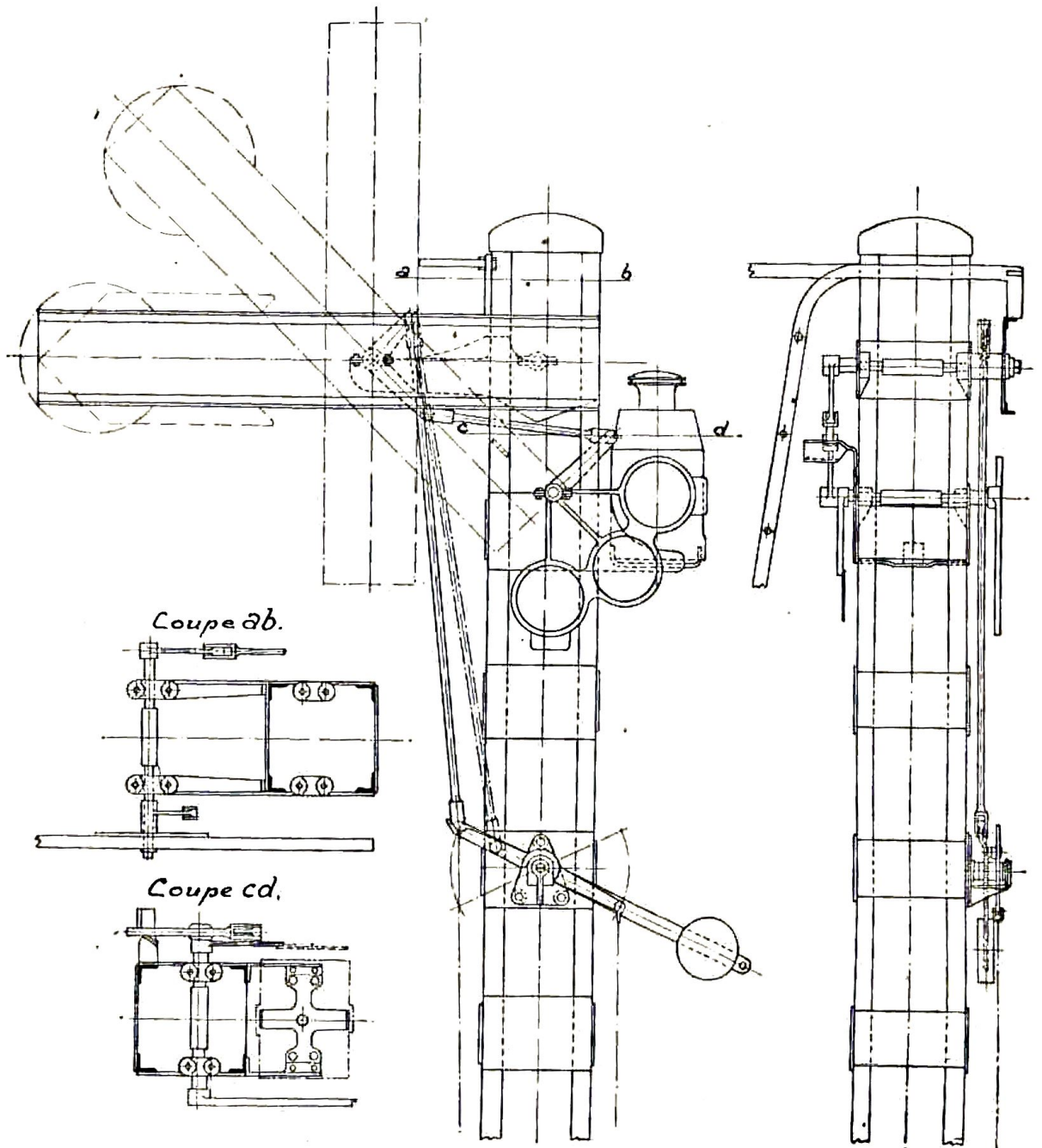
Fig. 72. — Sémaphore du nouveau type (État belge) à palette se levant verticalement (0-90°).
