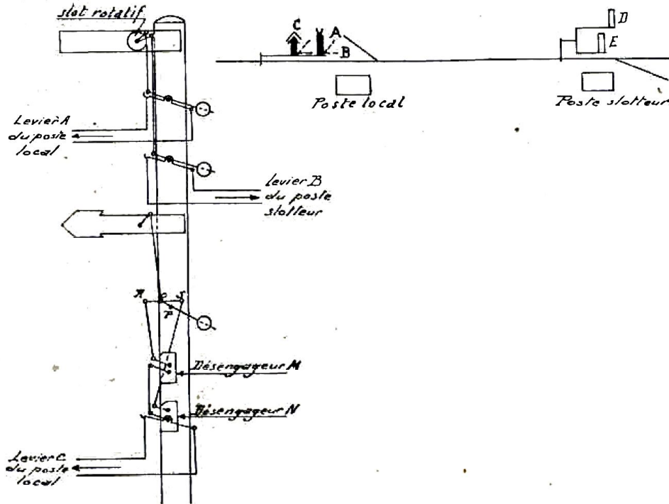
Fig. 109. — Schéma de la manœuvre d'une palette d'arrêt absolu à trois positions conjuguée avec une palette avertisseur à trois positions répétant les indications d'un chandelier de bifurcation.
