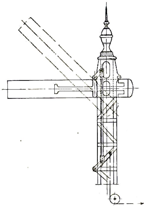
Fig. 32. — Sémaphore à palette levante manœuvrée à simple fil.
