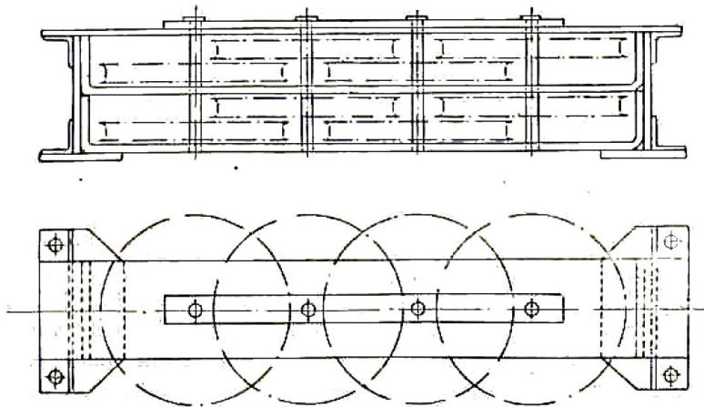
Fig. 45 — Châssis horizontal à deux étages et à huit poulies de renvoi de 300 mm.
