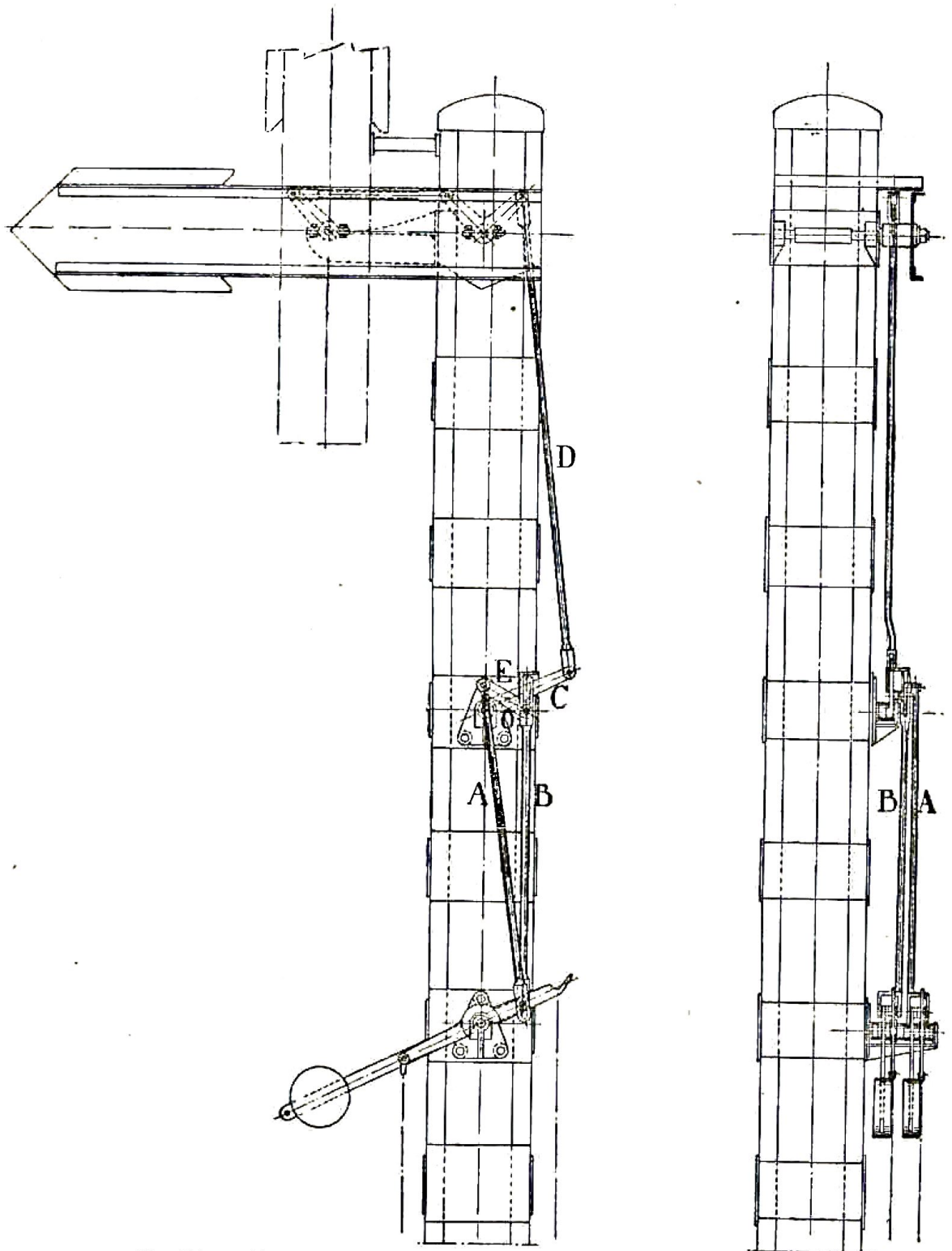
Fig. 76. -- Slot à coulisse monté sur un sémaphore à palette équilibrée.
