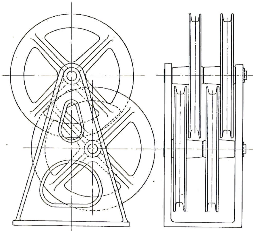
Fig. 41. — Support vertical à quatre poulies de renvoi de 300 mm.
