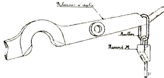
Fig. 59. — Raccord d'un fil au balancier à déclat réalisé au moyen d'un raccord M et d'un maillon fermé.
