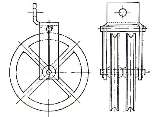
Fig. 47. — Poulie guide-fil.
