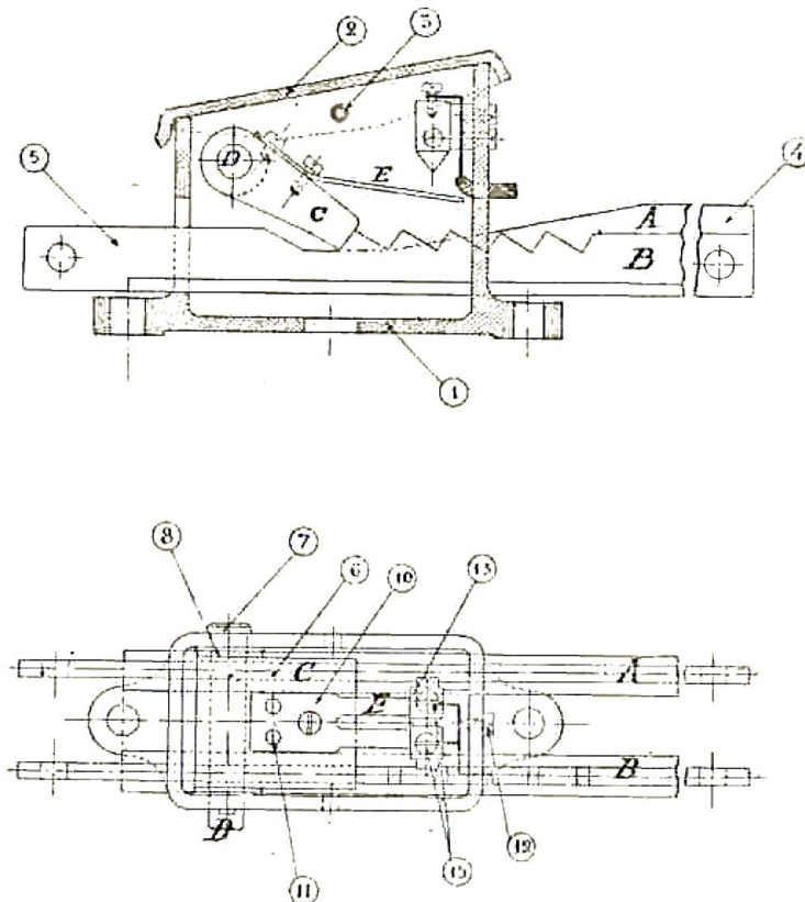
Fig. 86. — Taquet de slot système César.
