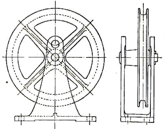
Fig. 40. — Support vertical à une poulie de renvoi de 300 mm.
