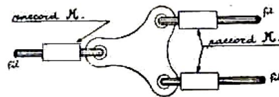
Fig. 61. — Assemblage de trois fils par un tréfle et trois raccords M.
