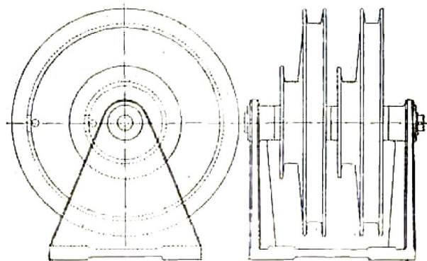
Fig. 70ter. Support vertical avec deux poulies différentielles.
