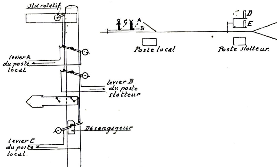
Fig. 108. — Schéma de la manœuvre d'une palette d'arrêt absolu à trois positions conjuguée avec une palette avertisseur se levant à 45° seulement.
