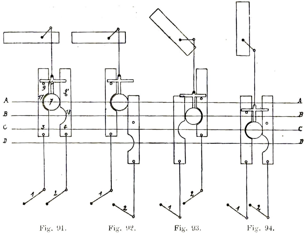
Fig. 91 à 94. — Schémas de la manœuvre du slot rotatif système César pour palettes à trois positions.
