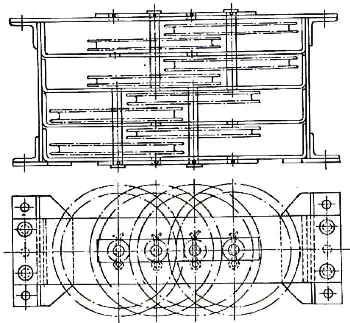
Fig. 46. — Châssis horizontal à quatre étages et à huit poulies de renvoi de 300 mm.
