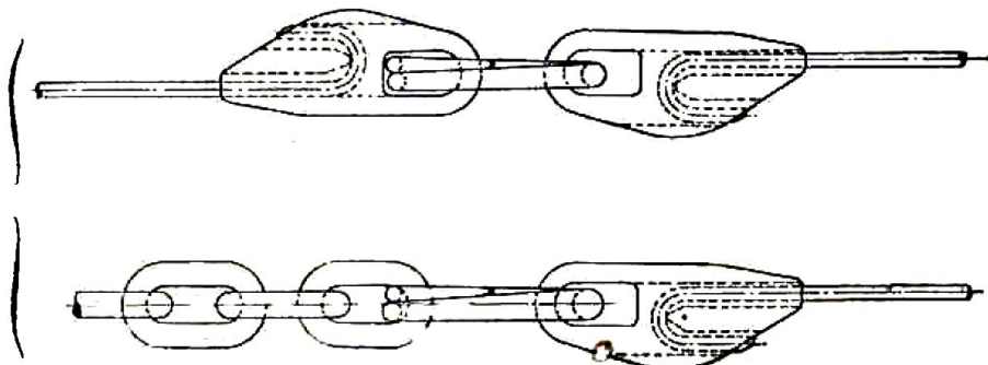
Fig. 49. — Assemblage de deux fils au moyen de deux raccords V et d'une fausse-maille, et assemblage d'un fil et d'une chaînette au moyen d'un raccord V et d'une fausse-maille.
