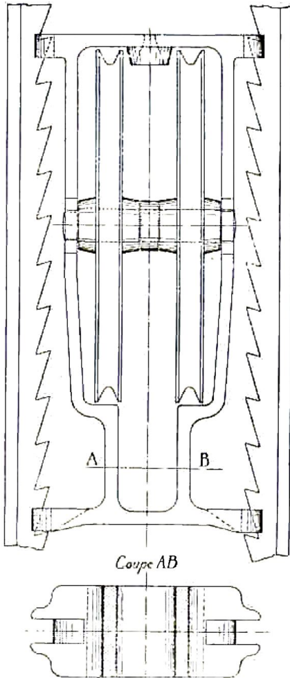
Fig. 66. L'étrier et les crémaillères du compensateur type État belge.
