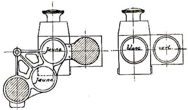
Fig. 74. — Trinocle et lanterne pour palette avertisseur 0-45°.
