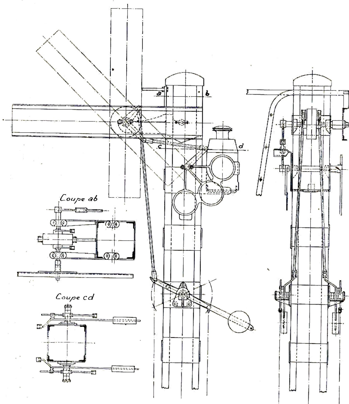
Fig. 96: — Sémaphore avec palette d'arrêt absolu à trois positions manœuvrée au moyen d'un slot rotatif système César monté derrière la palette sur l'arbre de rotation.
