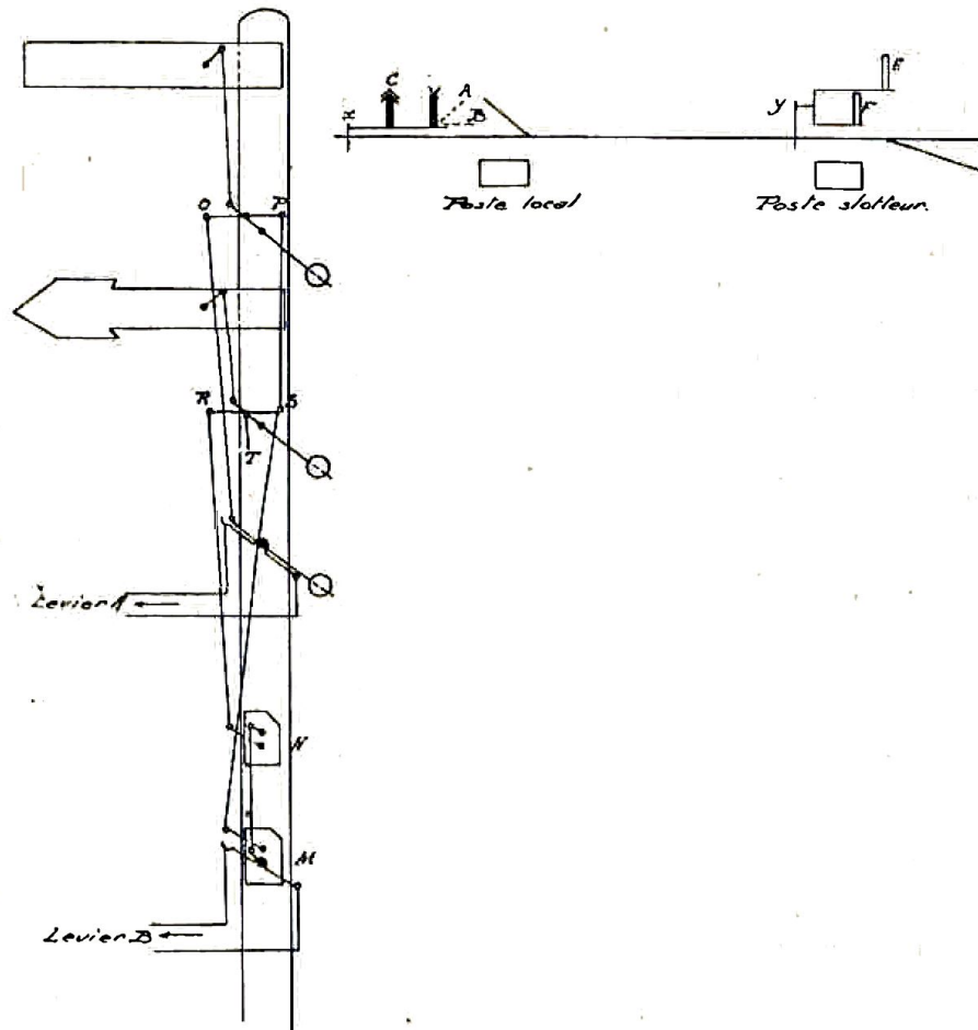
Fig. 111. — Schéma du nouveau dispositif pour la manœuvre d'une palette d'arrêt absolu à trois positions conjuguée avec une palette avertisseur à [trois] positions répétant les indications d'un chandelier de bifurcation.
