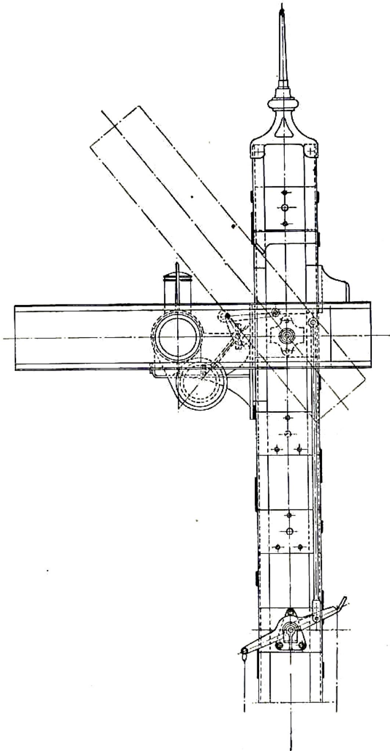
Fig. 71. — Sémaphore de l'ancien type (État belge) à palette se levant à 45°.
