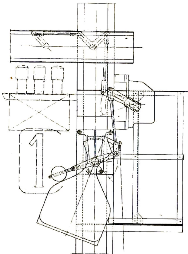
Fig. 104. — Slottage d'une palette à numéros réalisé au moyen d'un désengageur.
