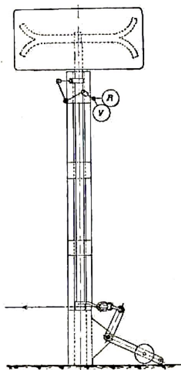
Fig. 30. — Signal à distance manœuvré à simple fil.
