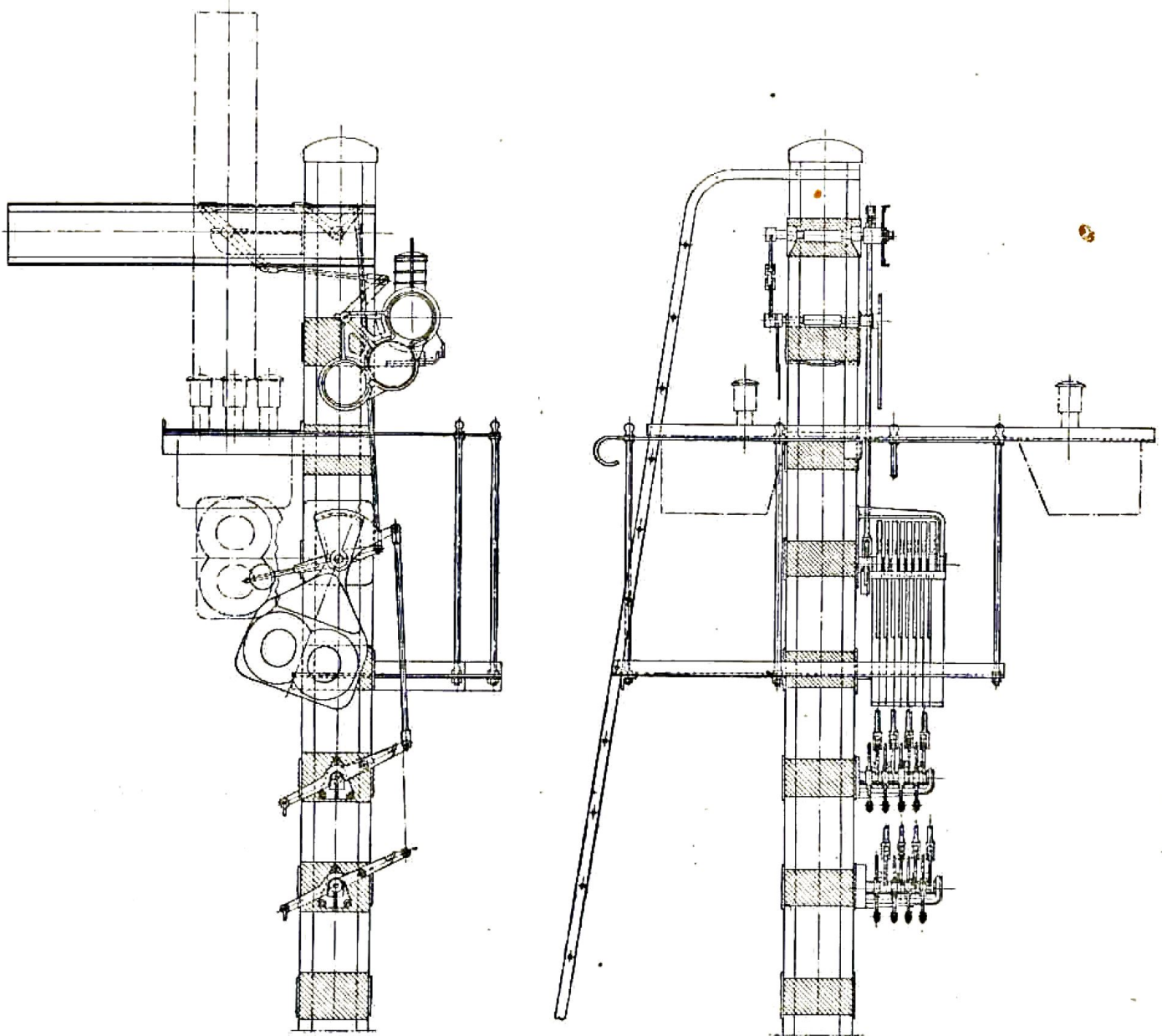
Fig. 103. — Palette équilibrée conjuguée avec huit numéros.
