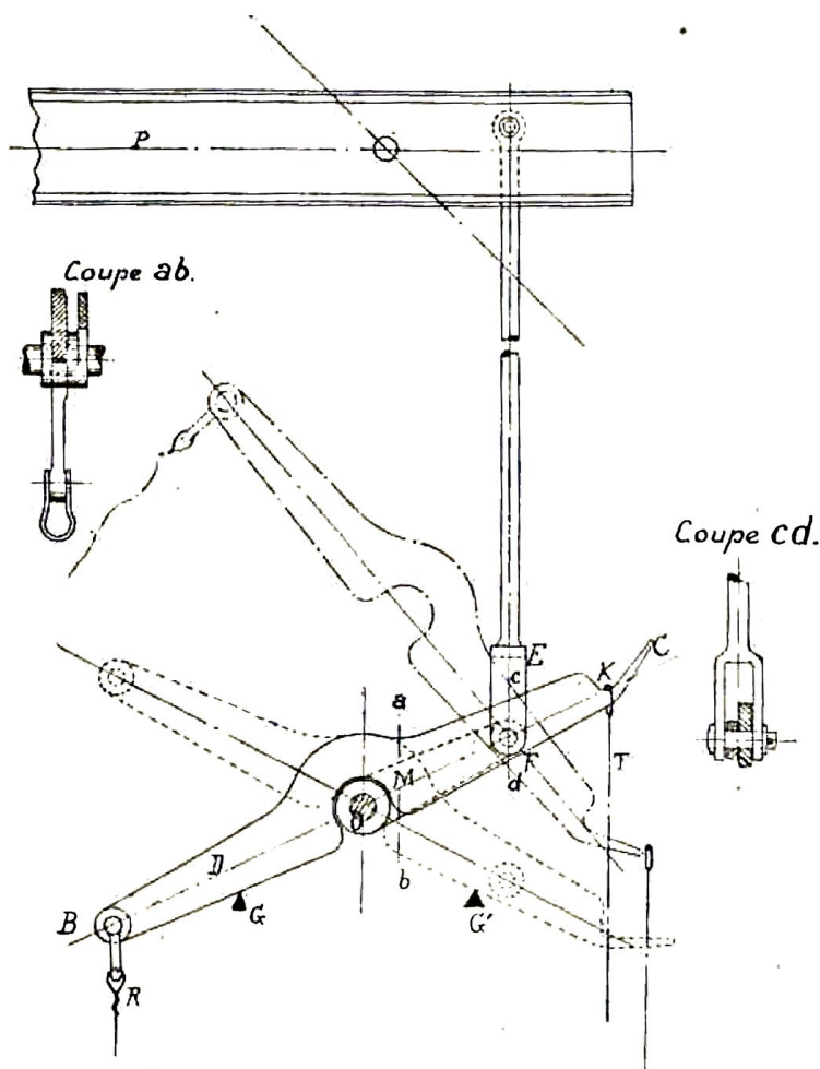
Fig. 34. -- Balancier à dé clic.
