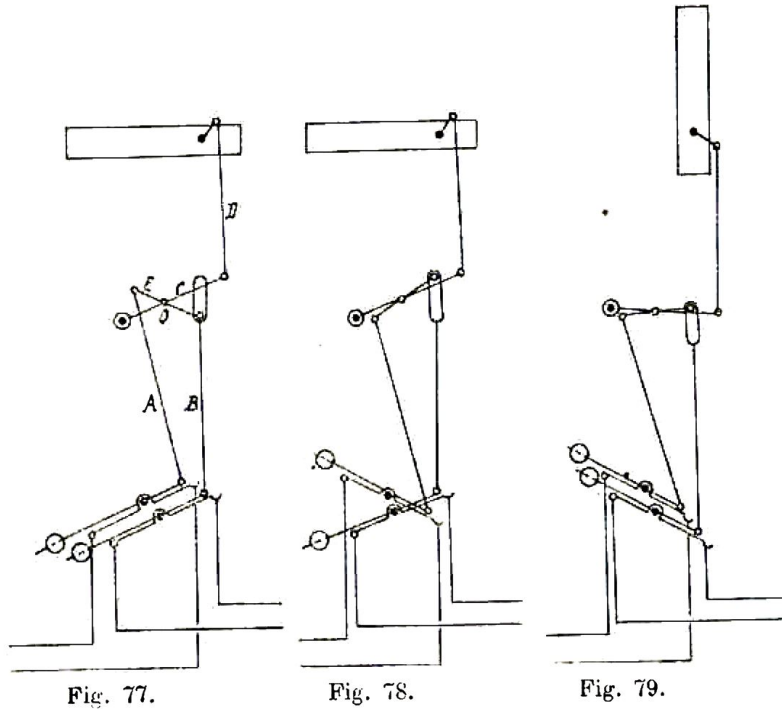
Fig. 77 à 79. — Schémas de la manœuvre du slot à coulisse.
