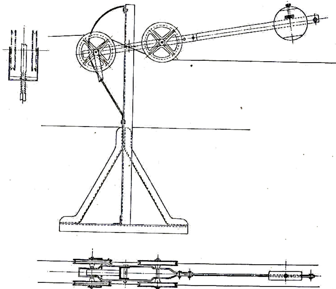
Fig. 68. — Compensateur allemand modifié.
