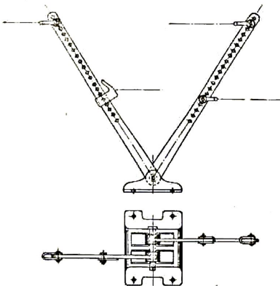
Fig. 70. — Balancier réducteur de course avec déclivité amovible.
