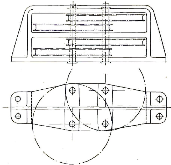
Fig. 44. — Châssis horizontal à deux étages et à quatre poulies de renvoi de 300 mm.
