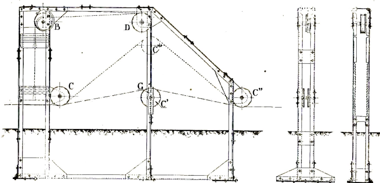
Fig. 63. — Compensateur type État belge.
