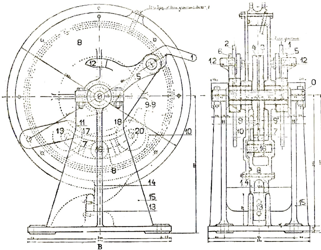
Fig. 83. — Slot rotatif système César.
