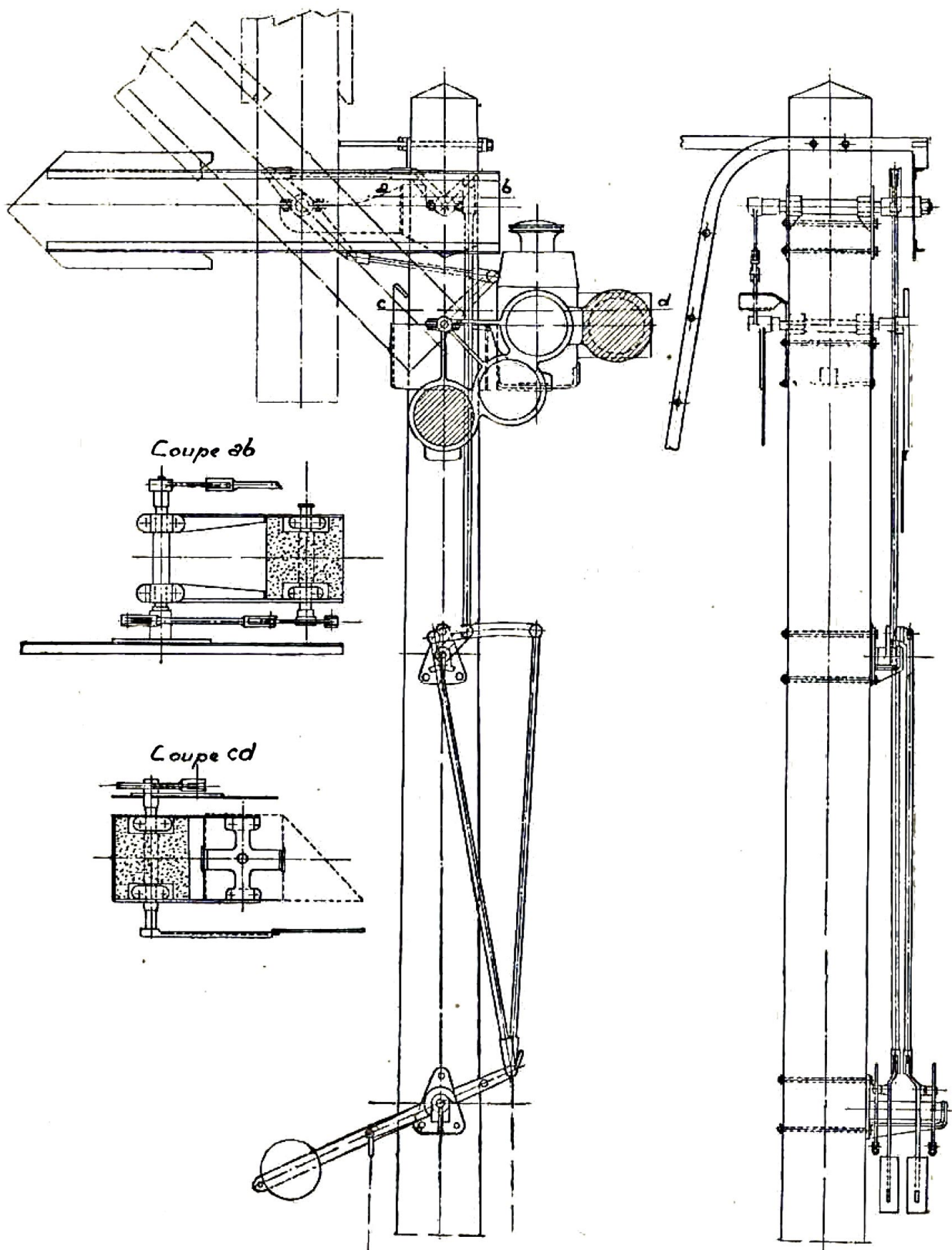
Fig. 102. — Palette avertisseur à trois positions montée sur un mât en béton armé et manœuvrée au moyen d'un balancier à bras inégaux.
